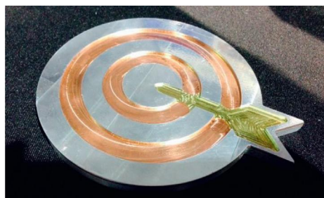
Рис. 9. Демонстрационный ММ образец возможности 3d-печати тремя материалами по технологии UAM (фото: Fabrisonic LLC, США)
