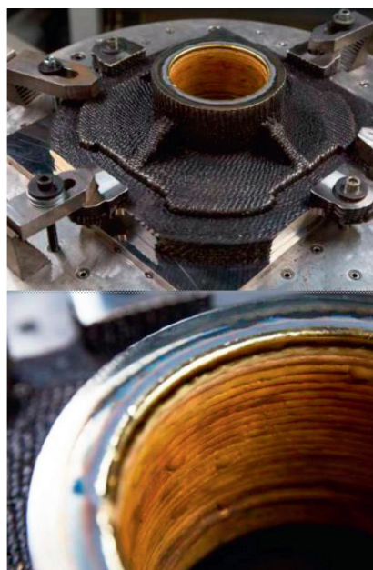
Рис. 6. ММ 3d-печать по технологии 3DMP/DED-W. (фото: Gefertec GmbH, FIT Additive Manufacturing Group, Германия)
