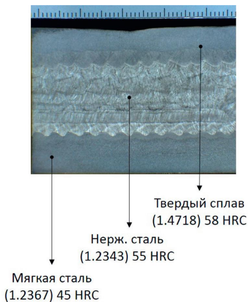
Рис. 6. ММ 3d-печать по технологии 3DMP/DED-W. (фото: Gefertec GmbH, FIT Additive Manufacturing Group, Германия)
