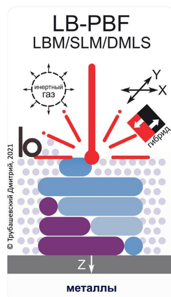
Рис. 13. Схема SLM технологии
